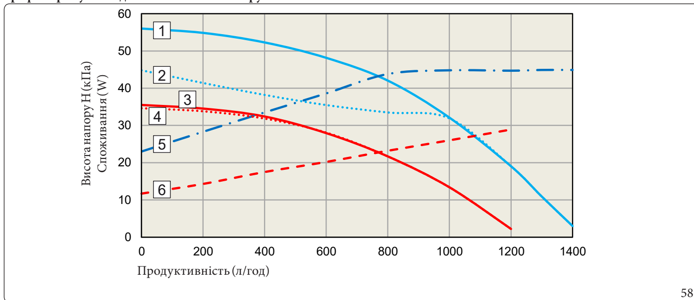
Графік Пропускна здатність - Висота напору - Споживання VICTRIX TERA V3 24 PLUSEU
