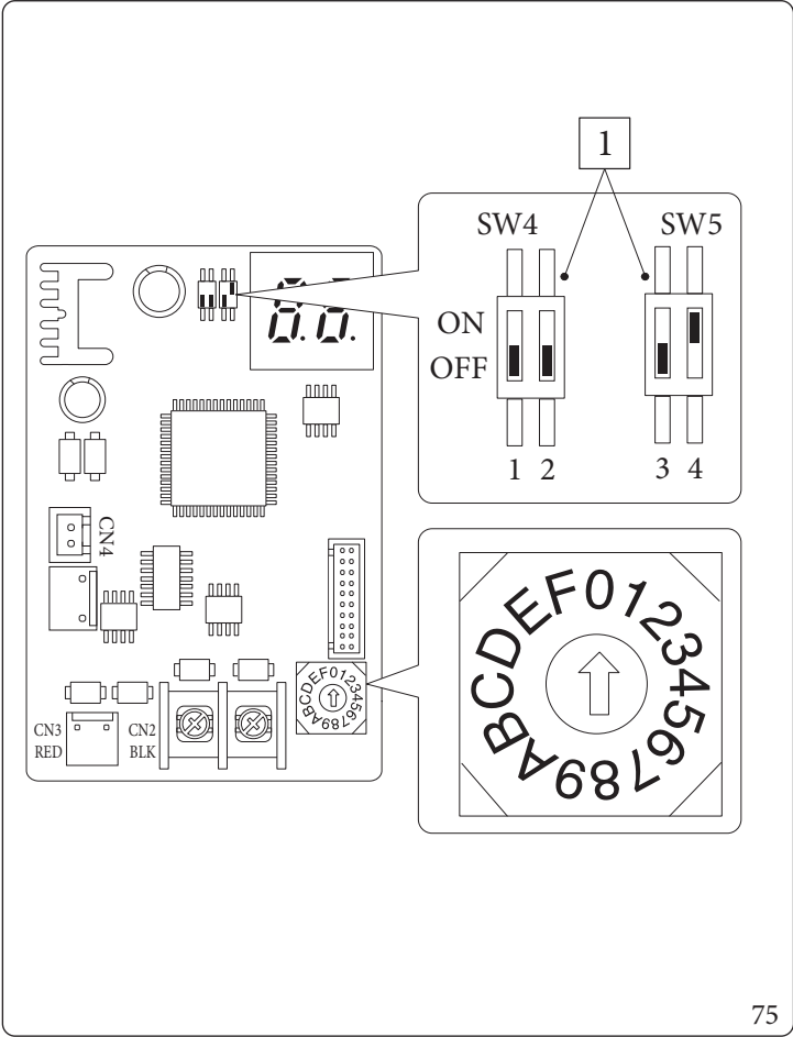
Умовні позначення (Мал. 75): 1 - Заводські настройки: не змінювати
