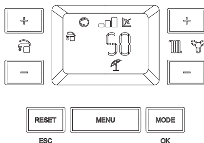
Режим Літо і процес нагрівання гарячої води
